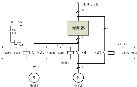
图3.3.3 一拖二变频1工频有软起模式
