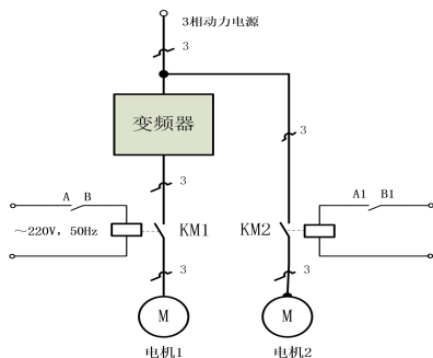
图3.3.2 一拖二变频1工频无软起模式
